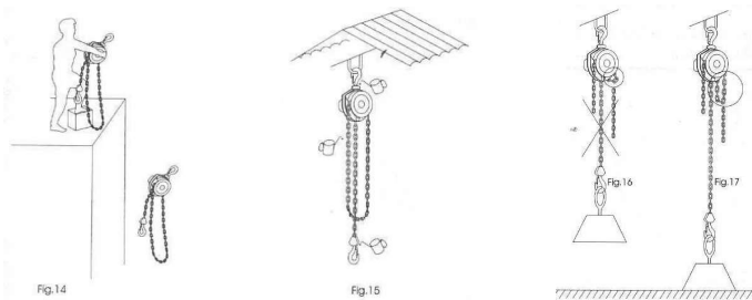
Figura 14 - Evitar maus tratos com equipamento, evitar joga-la, arrasta-la e etc. Figura 15 – Após o uso lubrificar a corrente de carga e todas as articulações dos ganchos, não lubrificar as lonas de freio, guardar o equipamento em local protegido.
