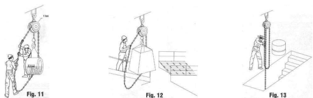
Figura 11 – Não sobrecarregar a talha. Antes de qualquer operação, verifique com segurança a carga a ser levantada (peso), para que se escolha o equipamento adequado (capacidade da talha). A carga jamais deverá ultrapassar a capacidade nominal da talha.
